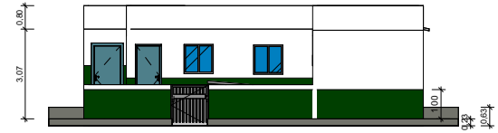
4 Fachada frontal 1 : 100
