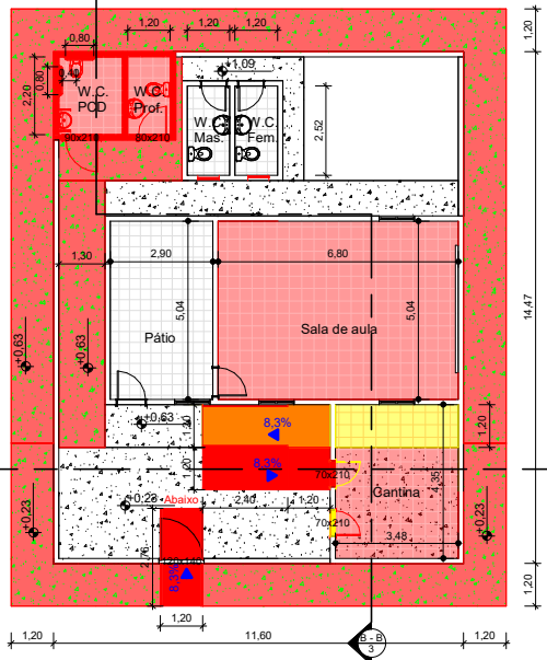
1 Térreo - Fase de reforma 1 : 100
