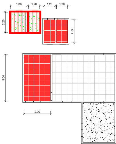
1 Térreo - Fase de reforma 1 : 100
